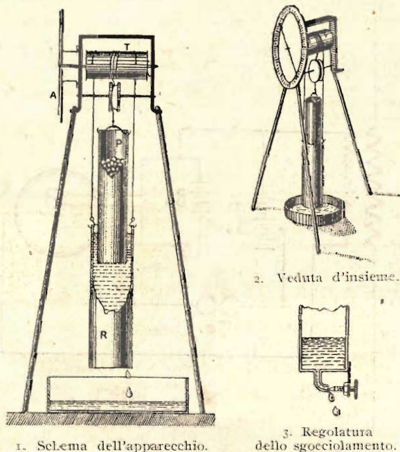
1. Schema dell'apparecchio.
